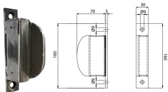
Knocker on column Klopfer an der Säule
