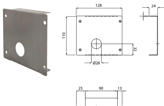
Lock cover Fußgängertor
