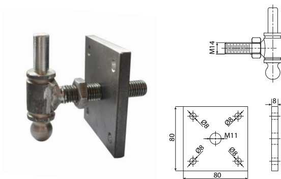
Hinge with wall plate Scharnier mit Wandplatte
